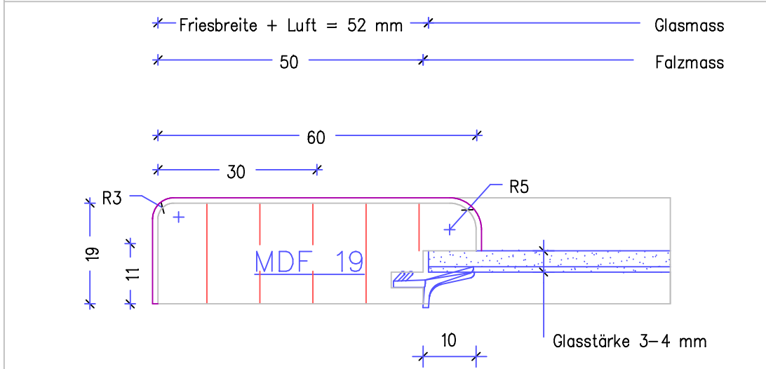
Schnitt A-A
