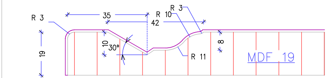
Schnitt C-C
