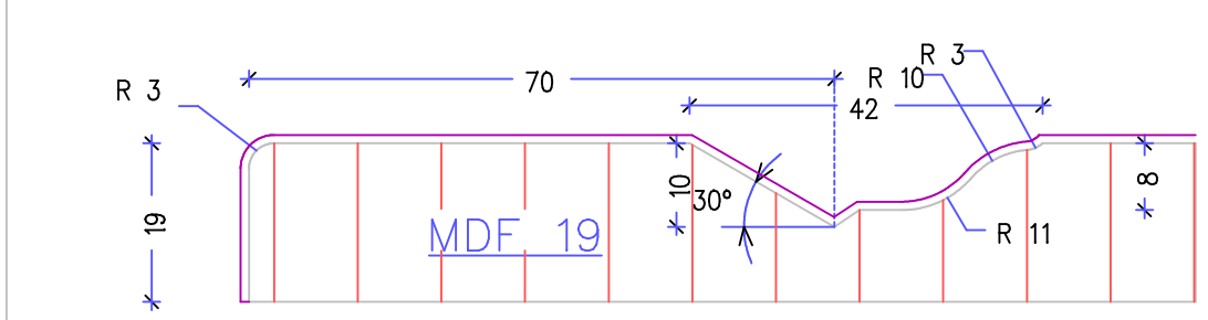
Schnitt A-A
